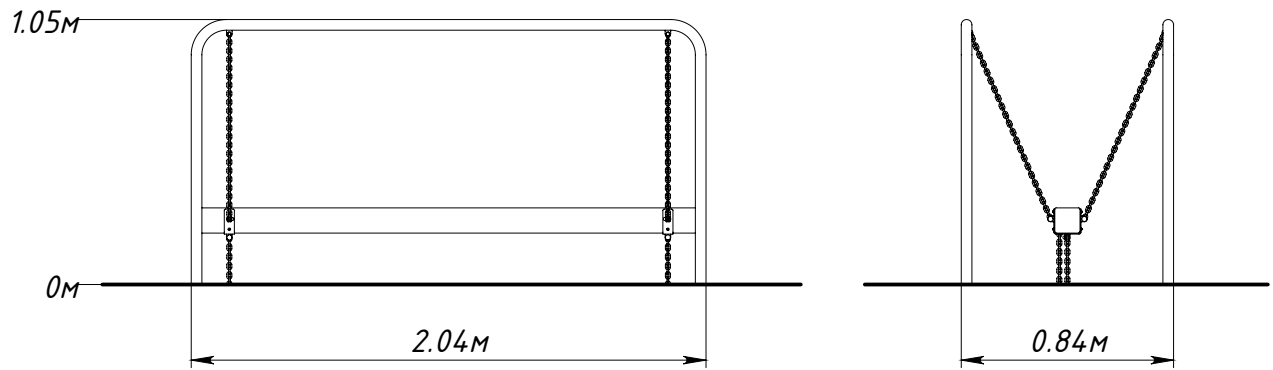
Рисунок 1 — Основные габаритные размеры
