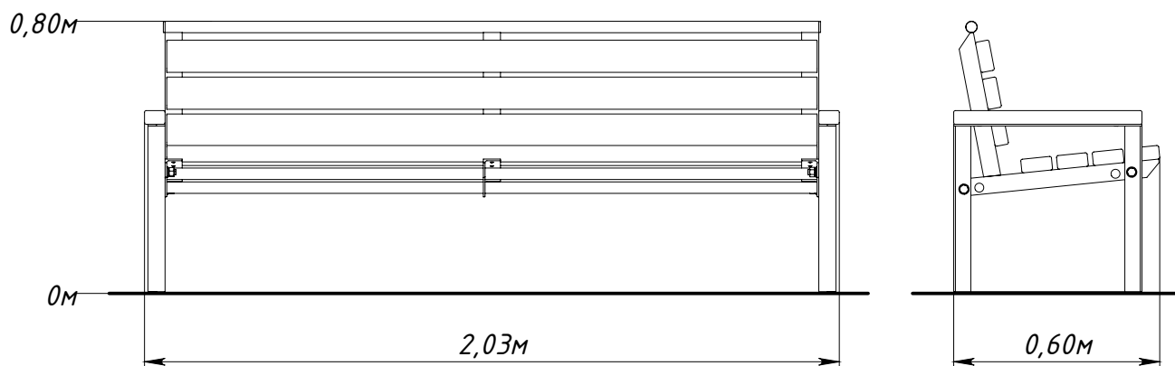
Рисунок 1 — Основные габаритные размеры
