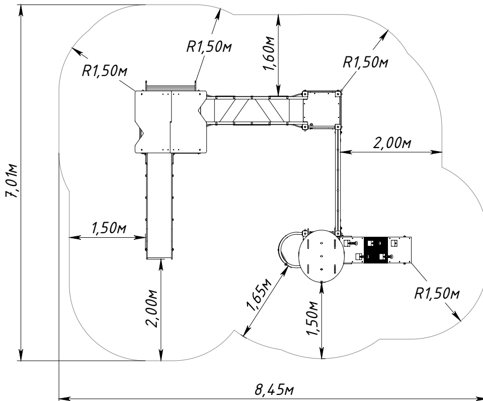
Рисунок 1 — Основные габаритные размеры
