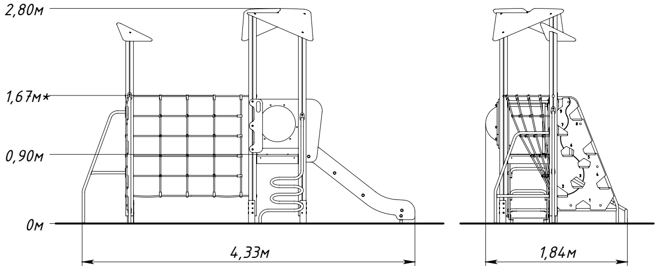
Рисунок 1 — Основные габаритные размеры
